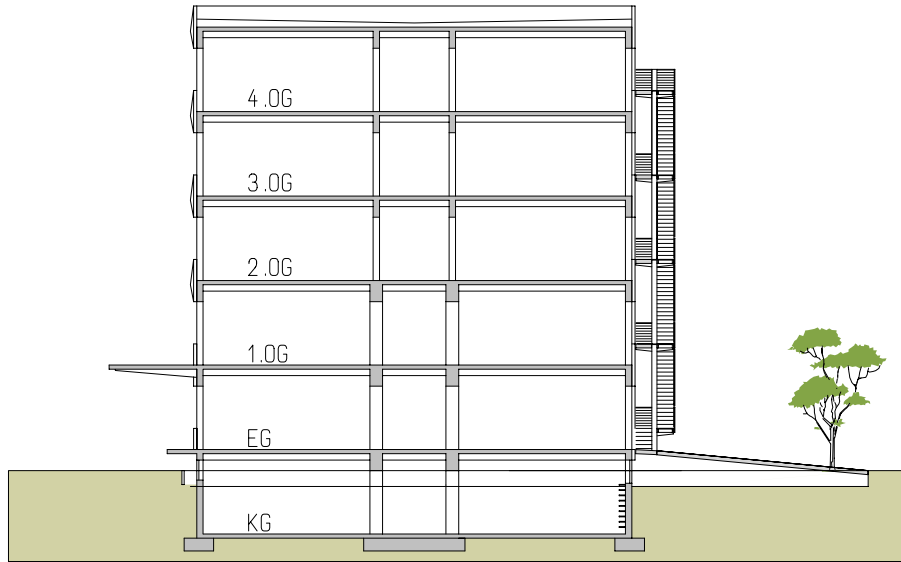
Schnitt Haus 11
