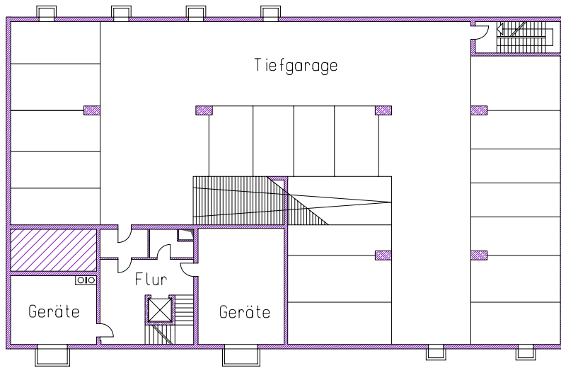
HAUS 11B 2.KELLERGESCHOSS
