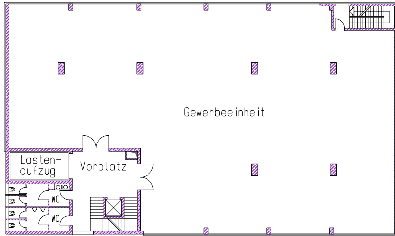
HAUS 11B 2.OBERGESCHOSS
