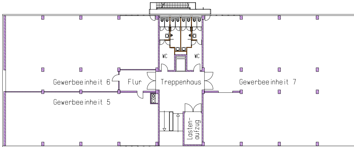
HAUS 11A 2.OBERGESCHOSS
