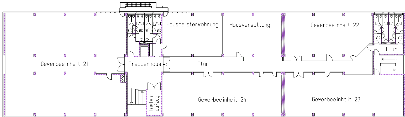
HAUS 11 4.OBERGESCHOSS
