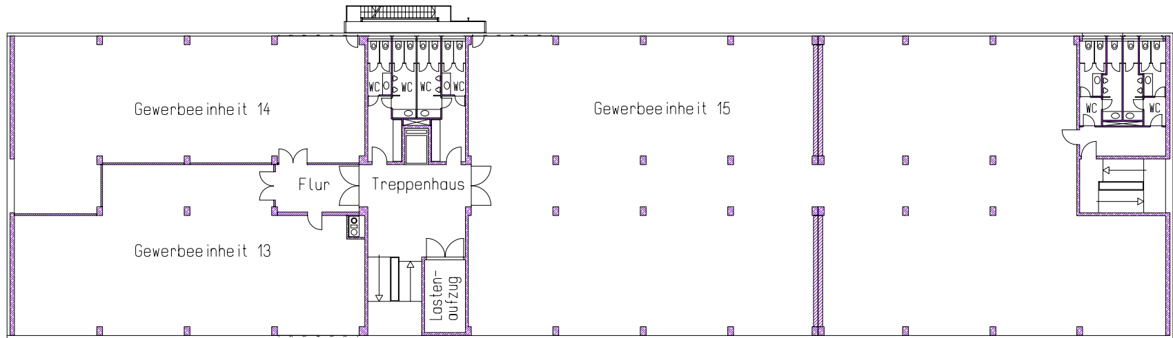
HAUS 11 2.OBERGESCHOSS
